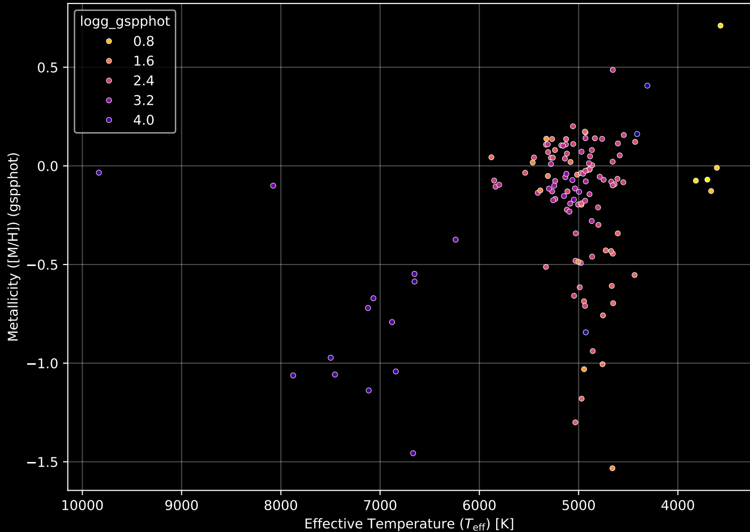
APOGEE DR17 Field: [000+14] Stellar Population Parameters (n= 131)
